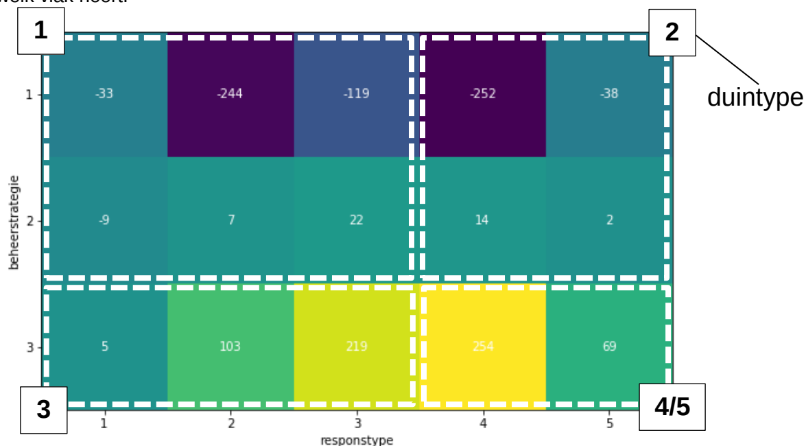
Figuur 3.7 Verschil in beheerstrategie, responstype en duintype tussen 2008 en 2017.
