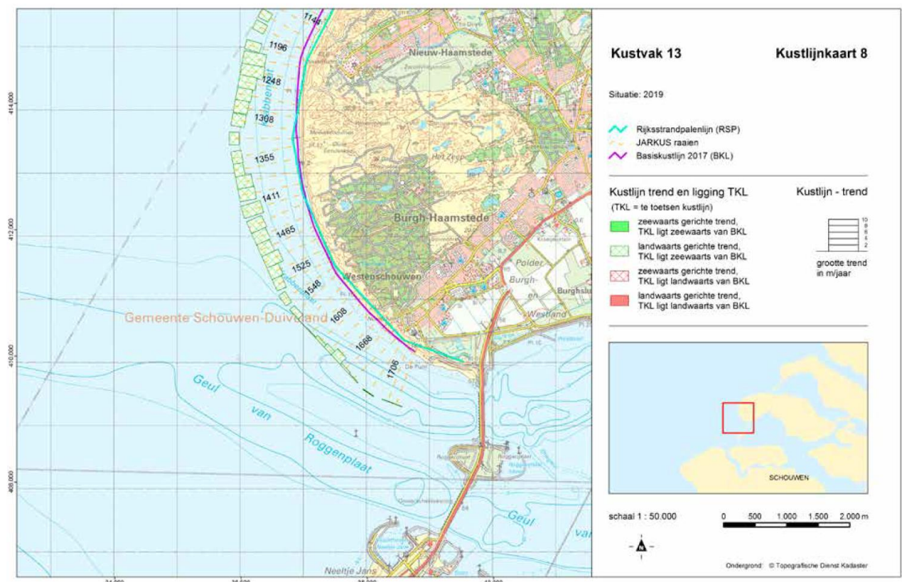
Figuur 6-5 Ligging studiegebied Schouwen (Kustlijnkaartenboek 2019). Het achteruitschrijden van de kust is zichtbaar uit de landwaartse trend van de MKL
