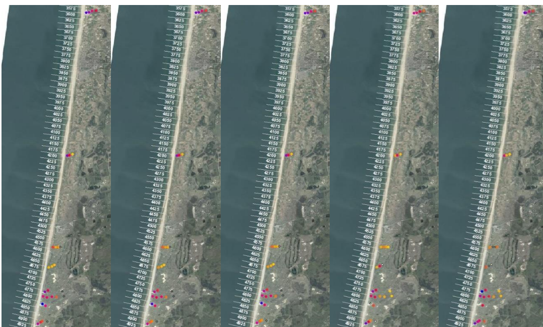
Figuur 6-4 Resultaten zandvangers. Van blauw via paars, rood, oranje naar geel zijn afnemende hoeveelheden gegeven. De figuren laten zien dat er een consistent patroon aanwezig is op plaatsen met een hoge dynamiek in de zeereep van zandtransport dat vele honderden meters landinwaarts gaat.
