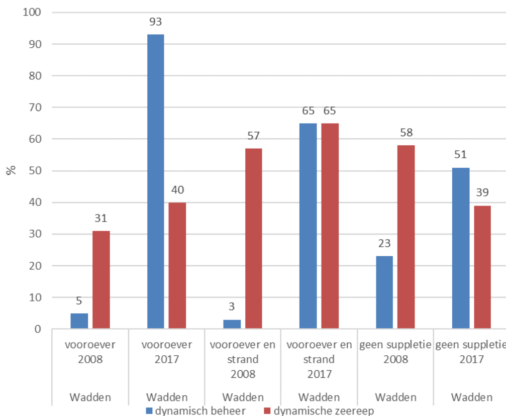
Figuur 5-4 Percentages Jarkusraai van de Wadden kust met een dynamisch beheer (beheerstrategie 3) en/of een dynamische zeereep (responstype 4 of 5).
