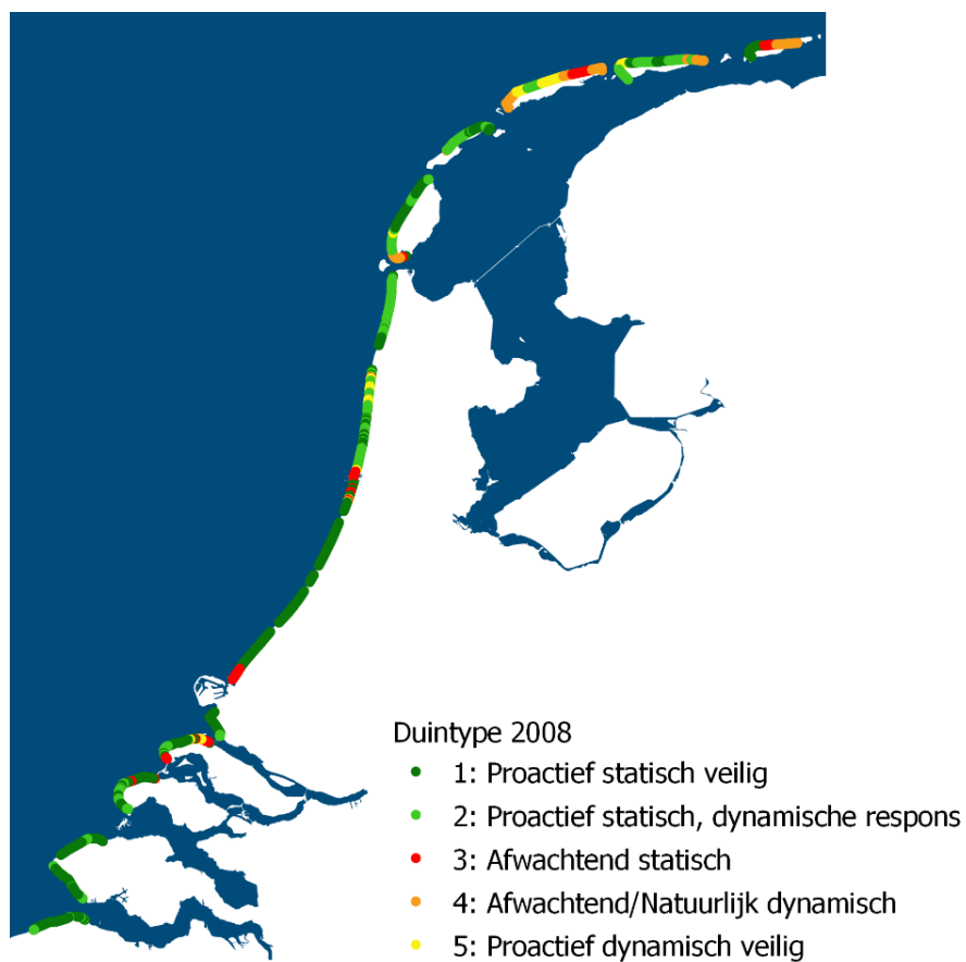
Figuur 3.1 Duintype verdeling van 2008 over de gehele Nederlandse kust, alle raaien meegenomen.
