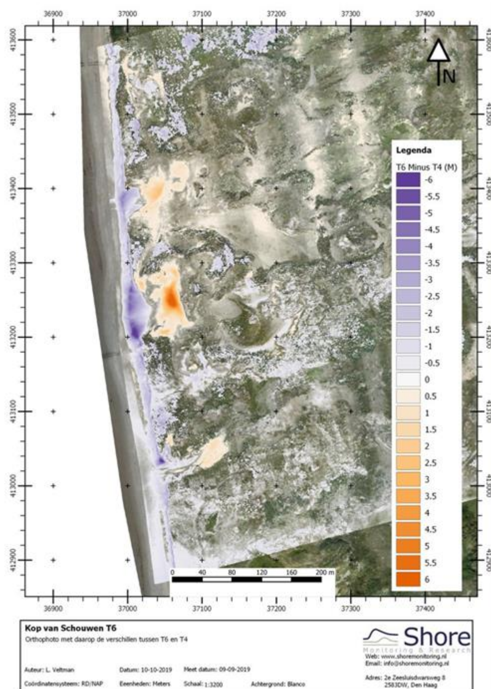
Figuur 6-7 overzicht van de hoogteveranderingen tussen T6 en T4 metingen (Shore, 2019). De bovenste twee ker- ven zijn de in september 2017 gegraven ker- ven; de onderste is een natuurlijk kerf. Let op de verschillen in morphologie.
