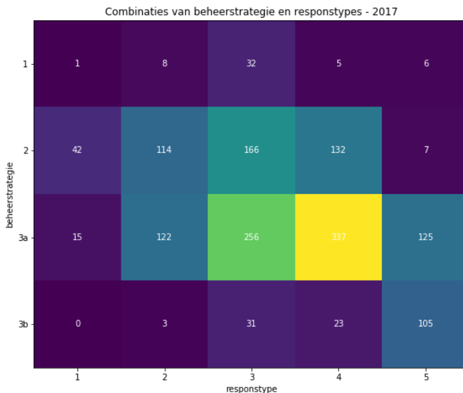
Figuur 3.6 Hittekaart van de combinaties van beheerstrategie en responstype in 2017.
