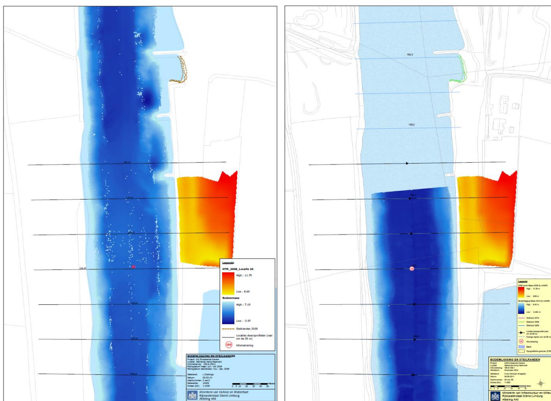
Figuur 3.24. Bodemligging en steilranden op de locatie Gebrande Kamp bij Neerveld in 2009 (links) en 2010 (rechts).
